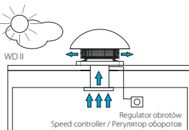
Montaż dachowy - wyciąg na zewnątrz budynku przy zastosowaniu zestawu montażowego. Roof installation - exhaust outside the building using the installation set. Монтаж на крышу - вытяжка наружу здания при помощи монтажного набора.
