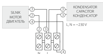
SCHEMAT PODŁĄCZENIA CONNECTION SCHEME / СХЕМА ПОДКЛЮЧЕНИЯ WD, WD II
