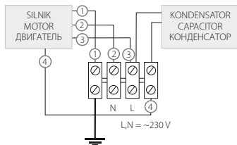
SCHEMAT PODŁĄCZENIA CONNECTION SCHEME / СХЕМА ПОДКЛЮЧЕНИЯ WD, WD II
