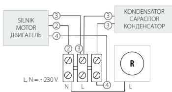
SCHEMAT PODŁĄCZENIA CONNECTION SCHEME / СХЕМА ПОДКЛЮЧЕНИЯ REGULATOR OBROTÓW SPEED CONTROLLER / РЕГУЛЯТОР ОБОРОТОВ EURO 0D
