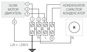
SCHEMAT PODŁĄCZENIA CONNECTION SCHEME / СХЕМА ПОДКЛЮЧЕНИЯ REGULATOR OBROTÓW / SPEED CONTROLLER / РЕГУЛЯТОР ОБОРОТОВ WD, WD II
