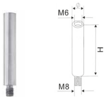
Pręt stały / Connect bar / прут постоянный
