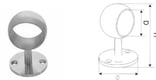
Wspornik ścienny poręczy / Handrail Support / стеновой держатель перил
