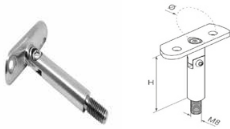
Pręt uchwyty poręczy z regulowaną blaszką montażową / Handrail support / прут зацепки перил с регулируемой монтажной пластинкой
