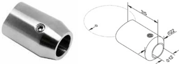
Uchwyt czołowy / Bar Holder / зацепка фронтальная
