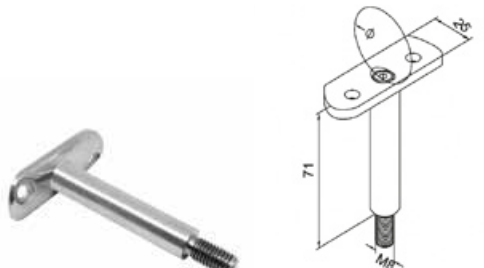
Pręt uchwyty poręczy z blaszką montażową / Handrail support / прут зацепки перил с монтажной пластинкой
