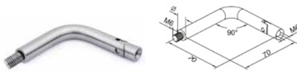
Kolanko regulowane z gwintem / Connect bar / регулирующее коленко с нарезкой
