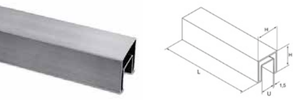
Pochwył nakładany / Applied handrail / наложенный перехват
