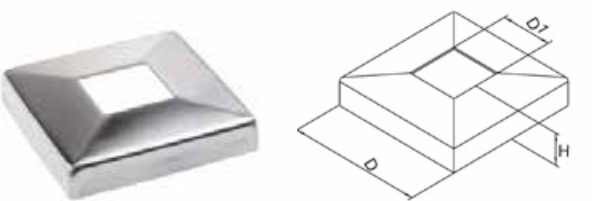
Rozeta maskująca / Base Cover / маскирующая розетка
