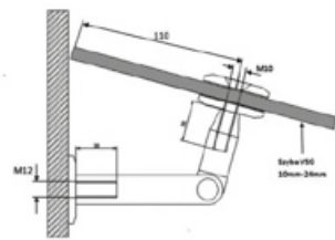
Uchwyt do daszku / Point fixing / зацепка к крыше
