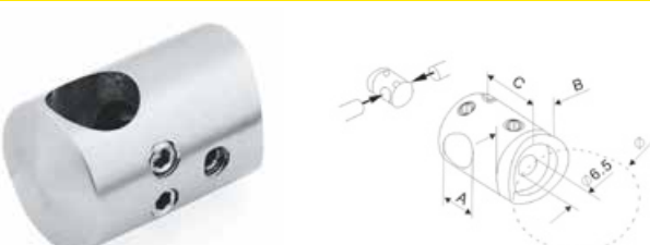
Uchwyt łączący pręty do rury / Bar holder / зацепка соединяющая стержень к трубе
