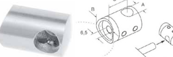
Uchwyt końcowy lewy do rury/ BHL Bar Holder Left / зацепка концевая левая к трубе
