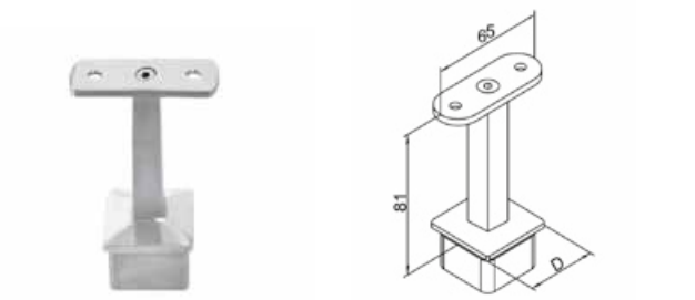
Łącznik poręczy / Handrail fitting / соединитель перил
