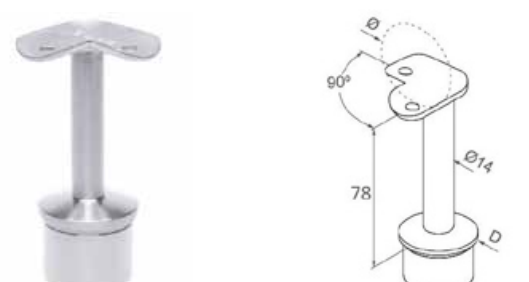
Podpora poręczy 90° / Handrail Support / подпорка перил
