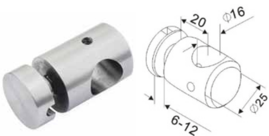
Uchwyt do szkła / Glass clamp / Зацепка для стекла
