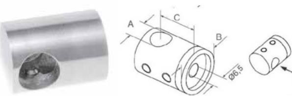
Uchwyt końcowy prawy do profilu / Bar Holder Right / ацепка концевая правая к профилю
