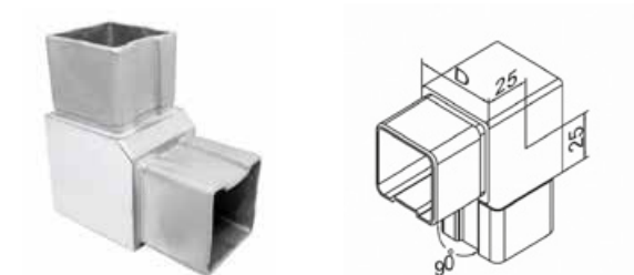
Łącznik pionowy / Vertical fitting / соединитель вертикальный
