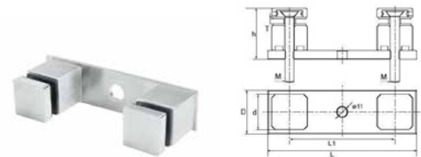
Uchwyt do szkła / Glass clamp / Зацепка для стекла
