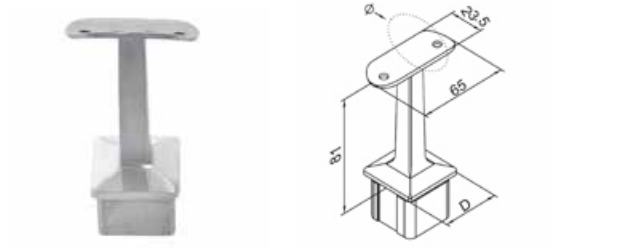
Łącznik poręczy / Handrail fitting / соединитель перил
