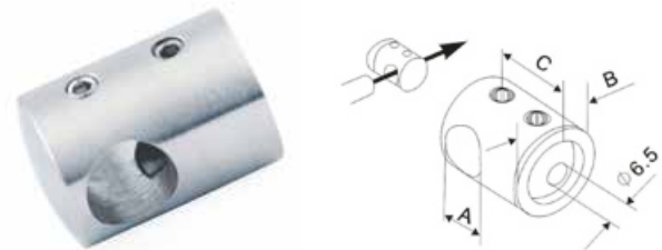
Uchwyt przelotowy pręta do profilu / Bar Holder / зацепка проходя стержня к профилю
