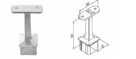
Łącznik poręczy / Handrail fitting / соединитель перил
