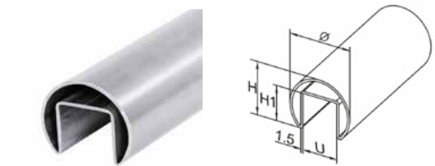
Pochwył nakładany / Applied handrail / наложенный перехват
