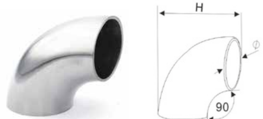
Kolanko do spawania / Flush Angle Weld / коленко для сварки
