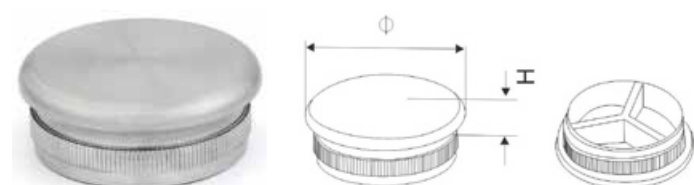
Zaślepka płaska pusta / End Cap Hollow / заглушка плоская пустая
