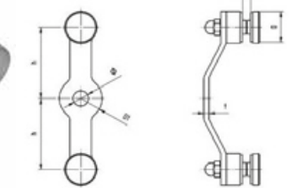
Uchwyt do szkła spider podwójny 180 / Spider clamp / зацепки к стеклу двойной
