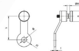
Uchwyt do szkła spider pojedynczy / Spider clamp / зацепки к стеклу единичные
