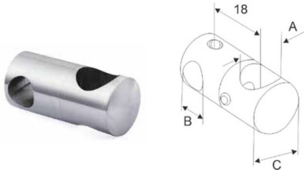
Uchwyt przelotowy pionowy / Bar Holder / зацепка проходная вертикальная
