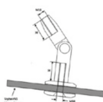
Uchwyt do daszku / Point fixing / зацепка к крыше
