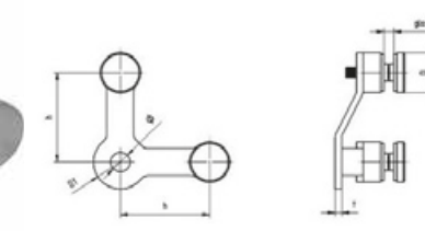
Uchwyt do szkła spider podwójny 90 / Spider clamp / зацепки к стеклу двойной
