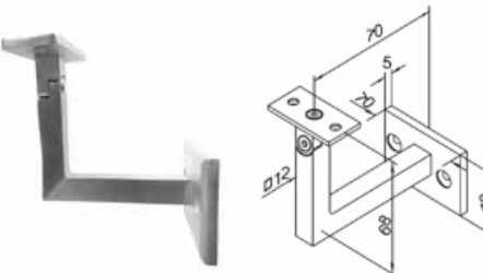
Uchwyt poręczy przegubowy / Handrail Bracket Adjustable / переломная зацепка перил
