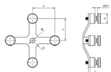
Uchwyt do szkła spider poczwórny / Spider clamp / зацепки к стеклу четвережный
