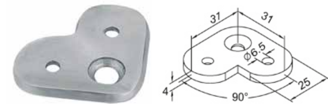
Blaszka montażowa 90° / Saddle / монтажная пластинка
