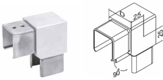
Łącznik pionowy / Vertical fitting / соединитель вертикальный
