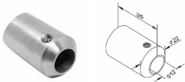
Uchwyt czołowy / Bar Holder / зацепка фронтальная
