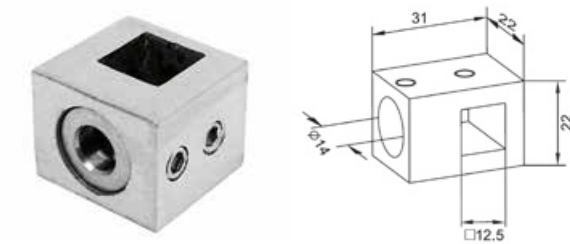
Uchwyt dla profilu / Bar Holder / зацепка для профиля
