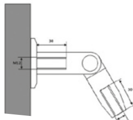
Uchwyt do daszku / Point fixing / зацепка к крыше
