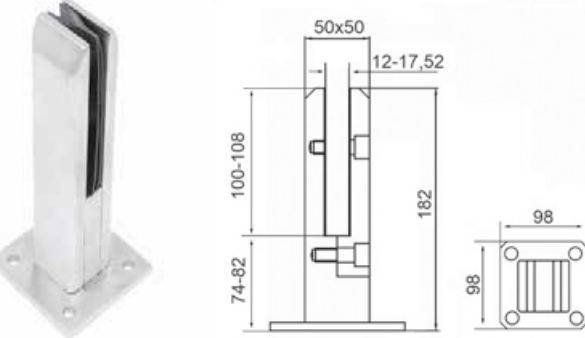
Uchwył podłogowy mocowanie szkła / Glass clamp / полая зацепкаприкрепляющая стекло
