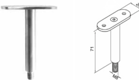
Pręt uchwyty poręczy z blaszką montażową / Handrail support / прут зацепки перил с монтажной пластинкой
