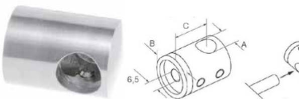
Uchwyt końcowy lewy do profilu / BHL Bar Holder Left / зацепка концевая левая к профилю
