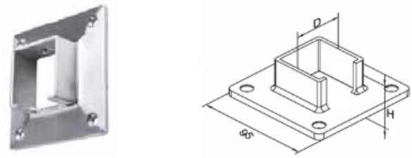
Osiowe mocowanie poręczy / Wall and bottom handrail fastenning / осевое прикреплeние перил
