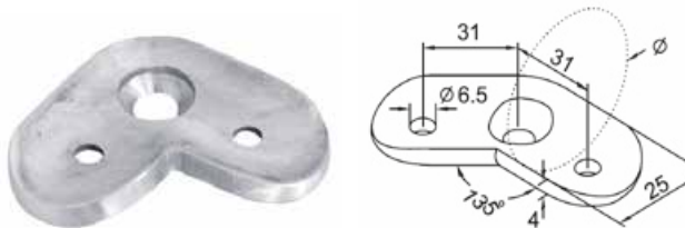
Blaszka montażowa 90° / Saddle / монтажная пластинка
