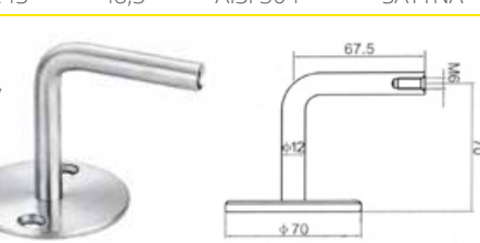
Uchwyt poręczy / Handrail Bracket / зацепка перил
