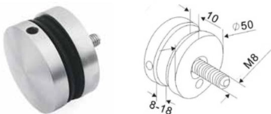
Punktowy uchwyt do szkła / Glass holder / пунктовая зацепка к стеклу
