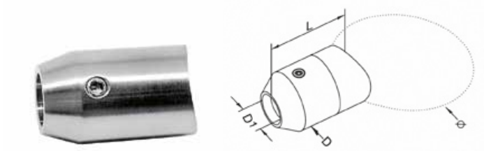
Uchwyt przelotowy linki / Rope crossbar holder / Переломная зацепка каната
