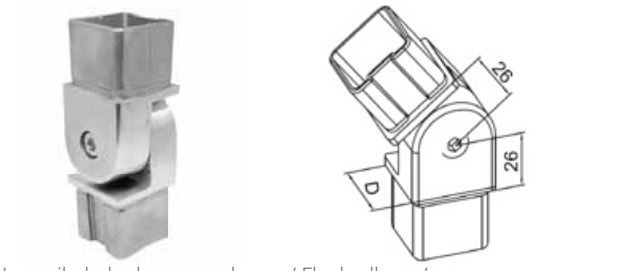
Łącznik- kolanko przegubowe / Flush elbow / регулирующее коленко
