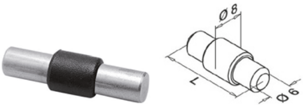
Sworznie zabezpieczające / Security Pin for Glass Clamp/ обезпечивающий стержень
