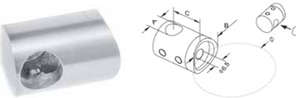
Uchwyt końcowy prawy do rury / Bar Holder Right / ацепка концевая правая к трубе
