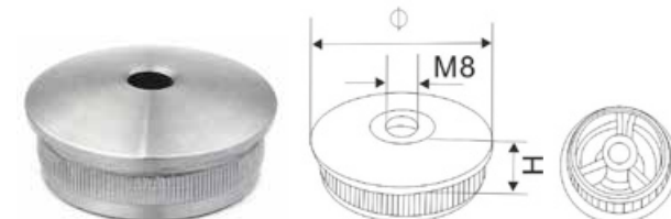
Zaślepka wypukła wbijana / End Cap / заглушка выпуклая вбитая
