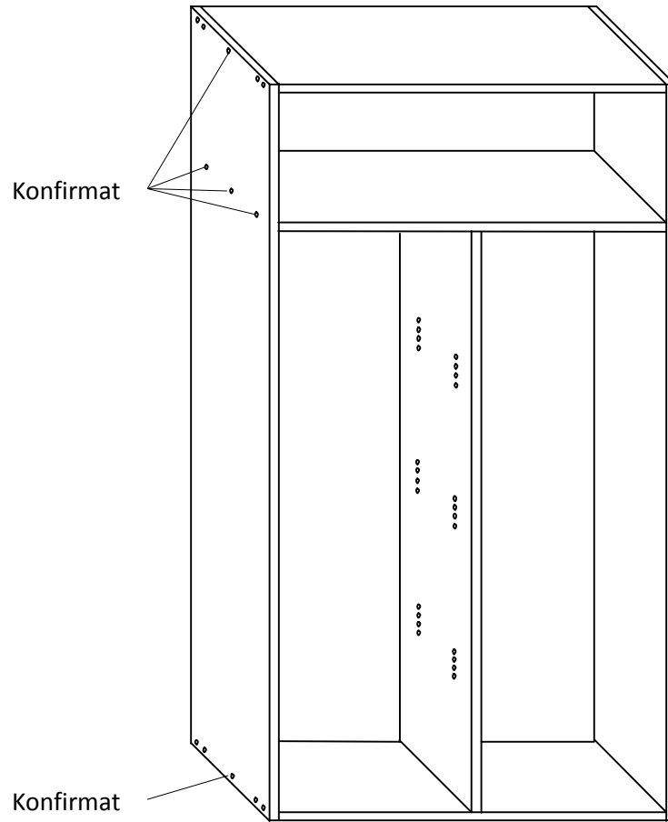
1 – Montaż korpusu
