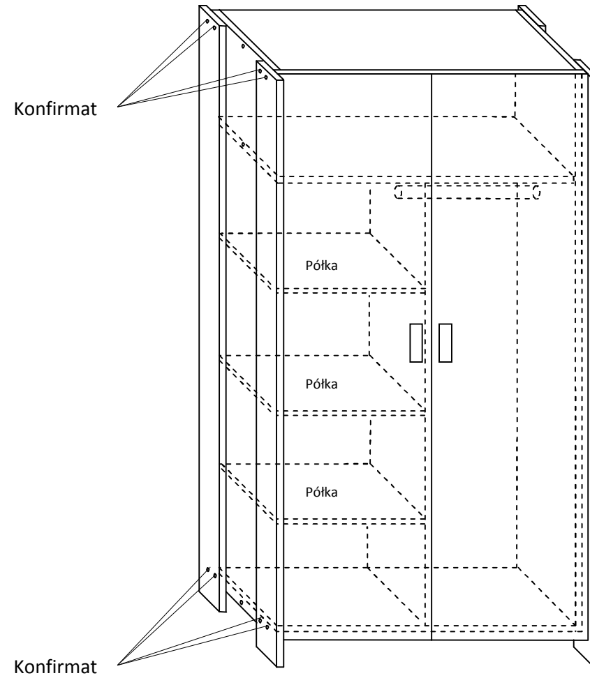
2 – Montaż w całość
