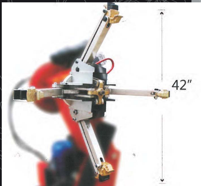
Uchwyt samo centrujący
