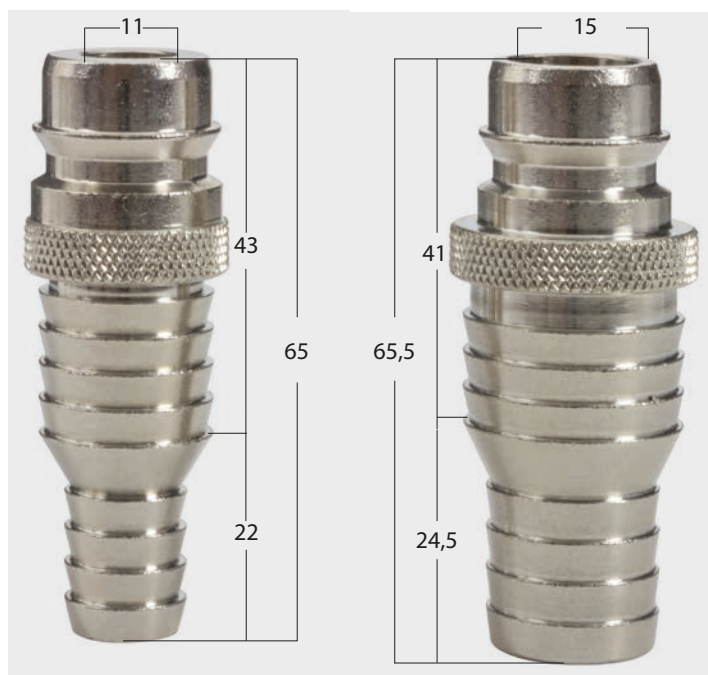
ST-45. Szybkozłącze : 3/4" GW
